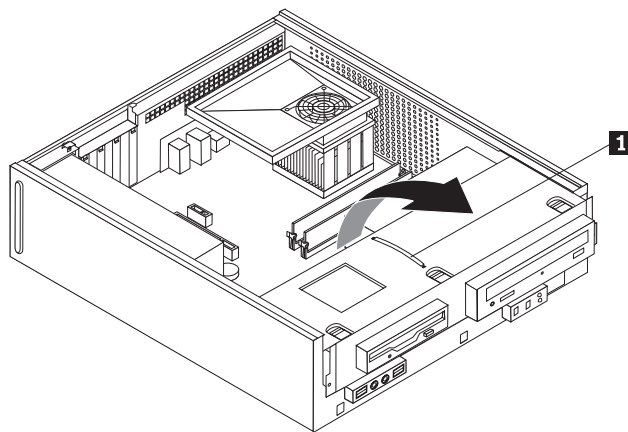
Σχήμα 8. Αφαίρεση του τμήματος τοποθέτησης μονάδων
