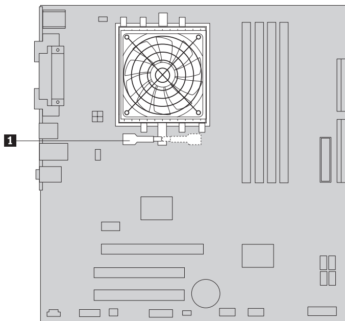
Σχήμα 31. Στερέωση της ψύκτρας με σφιχτήρα στο πλαστικό πλαίσιο συγκράτησης
