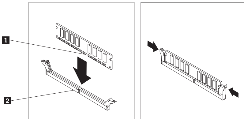
Σχήμα 10. Τοποθέτηση της μονάδας μνήμης
