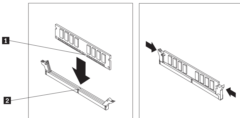
Figur 10. Plassering av minnemodulen
