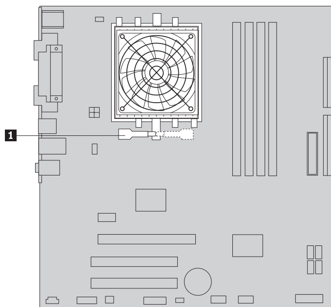
Figur 31. Klemme fast kjøleribben til støttebraketten i plast
