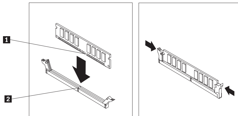
Figura 10. Posicionar o módulo de memória
