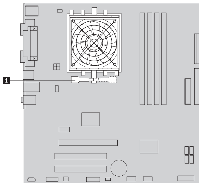
Figura 31. Fixar o dissipador de calor com um grampo ao suporte de fixação de plástico
