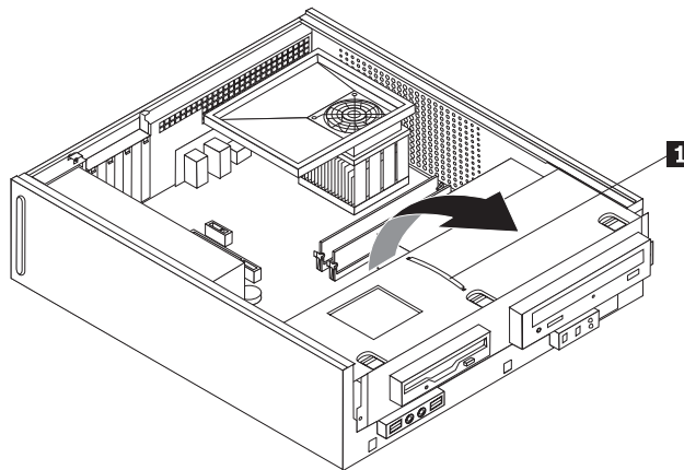
Figura 8. Remover o conjunto dos compartimentos de unidades
