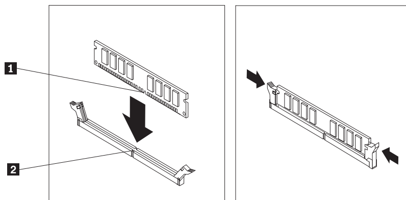
Figura 34. Instalar o módulo de memória
