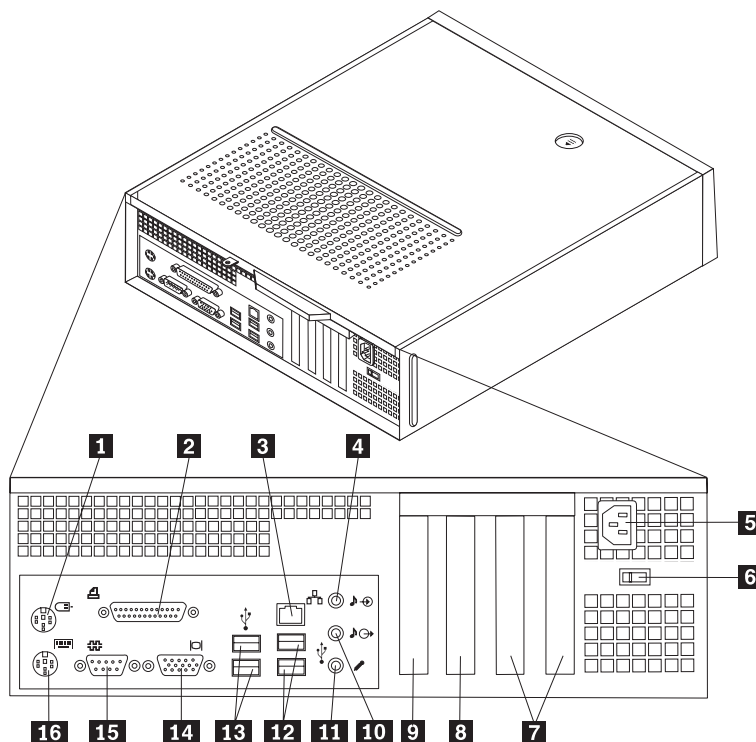
Figura 2. Localizações de conectores
