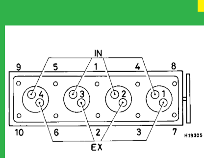
1360 cm 3 , TU3
