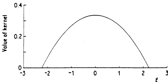
Fig. 79 Epanechnikov kernel.
