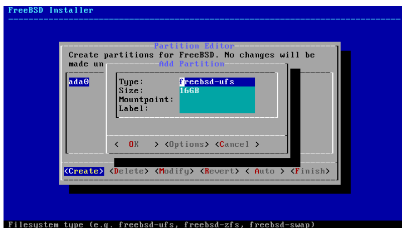
Abbildung 2.19. Partitionen manuell erzeugen
