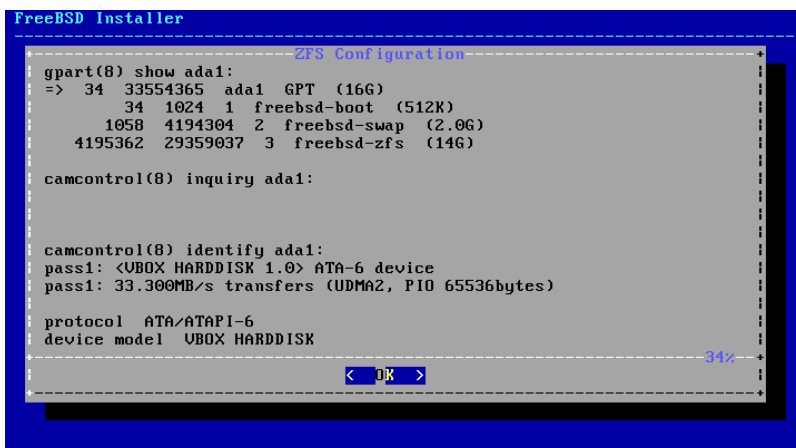
Abbildung 2.25. Informationen zum Laufwerk
