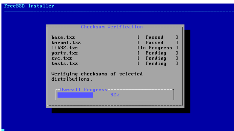
Abbildung 2.32. Überprüfen der Distributionsdateien
