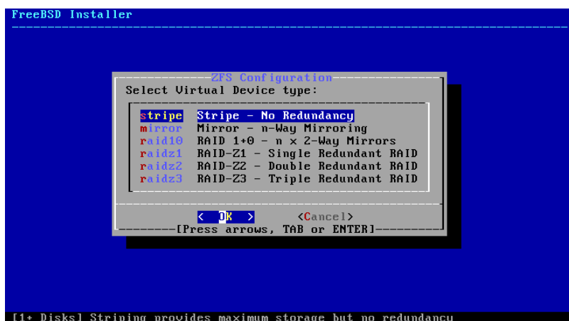
Abbildung 2.21. ZFS Pool Typen
