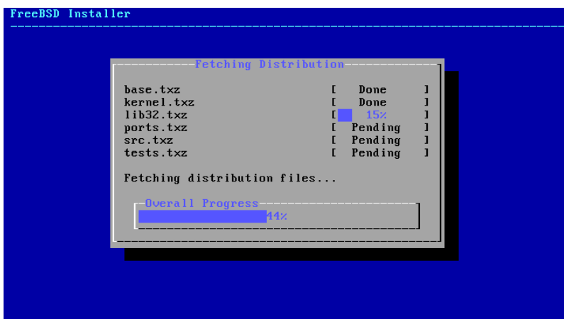
Abbildung 2.31. Herunterladen der Distributionsdateien
