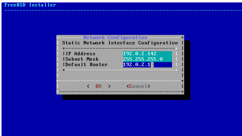
Abbildung 2.55. Statische IPv4-Konfiguration
