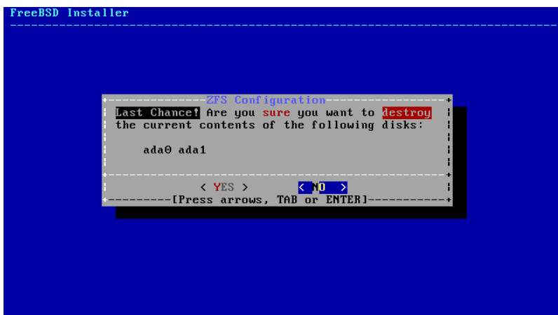
Abbildung 2.28. Letzte Chance!
