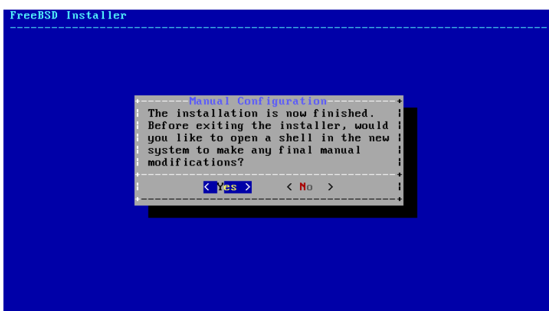
Abbildung 2.47. Manuelle Konfiguration
