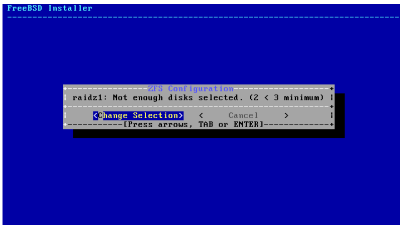
Abbildung 2.23. Ungültige Auswahl
