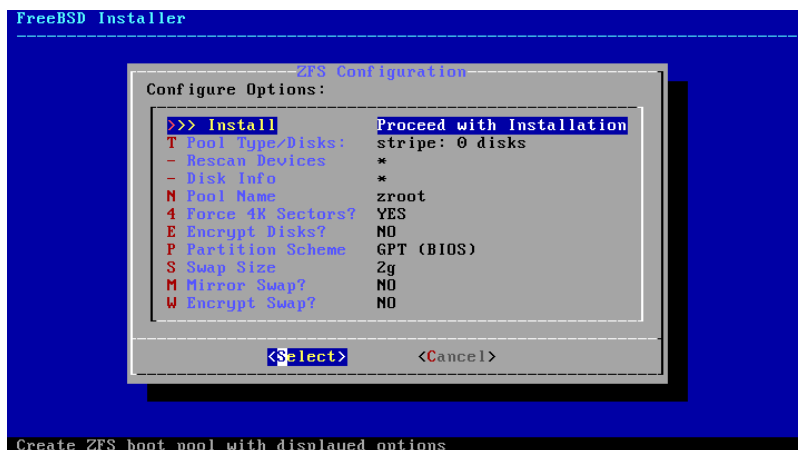
Abbildung 2.20. ZFS Konfigurationsmenü
