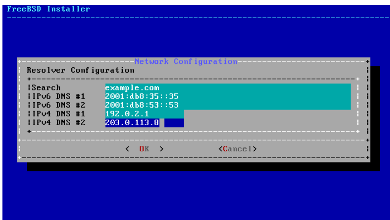
Abbildung 2.59. DNS-Konfiguration
