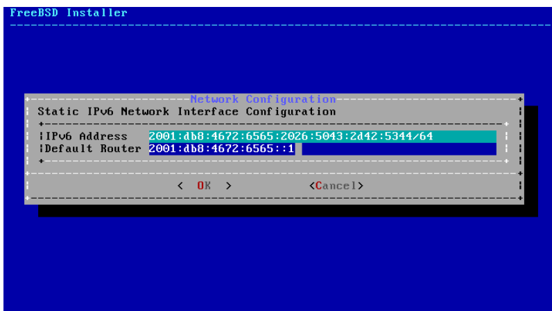
Abbildung 2.58. Statische IPv6-Konfiguration
