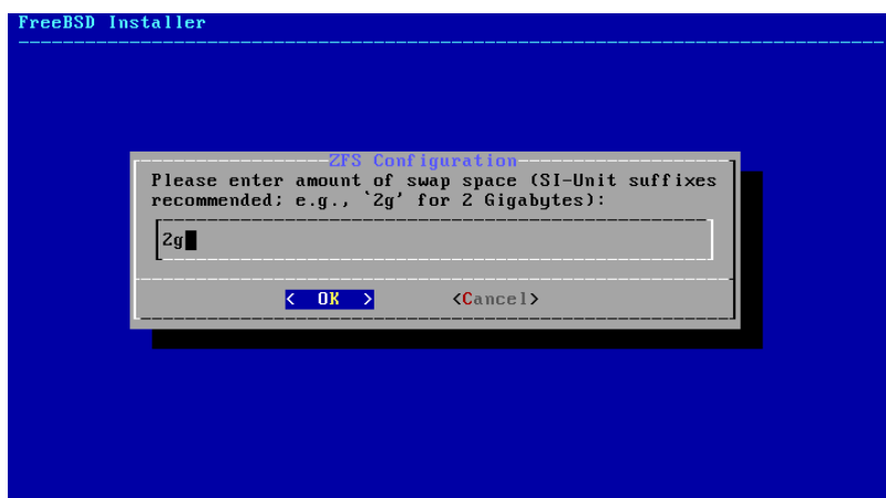
Abbildung 2.27. Größe des Swap-Speichers
