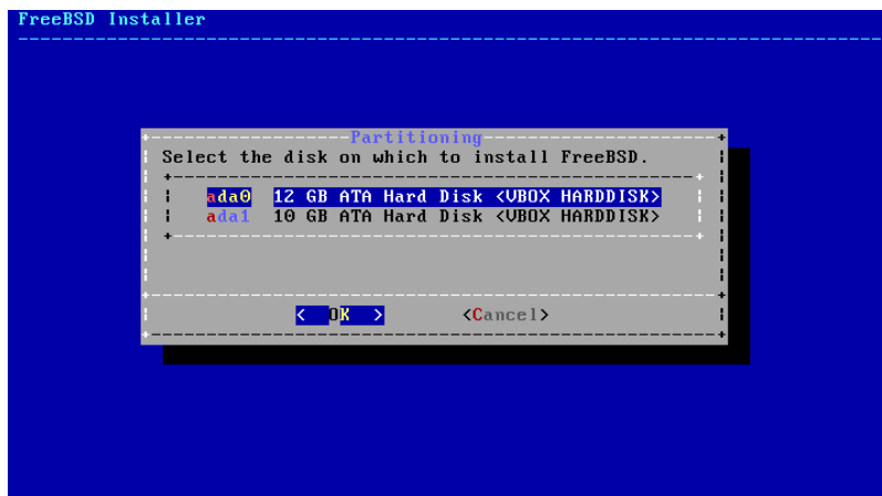
Abbildung 2.11. Aus mehreren Platten eine auswählen
