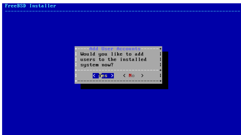
Abbildung 2.43. Benutzerkonten hinzufügen
