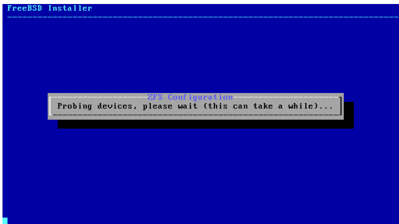
Abbildung 2.24. Rescan Devices
