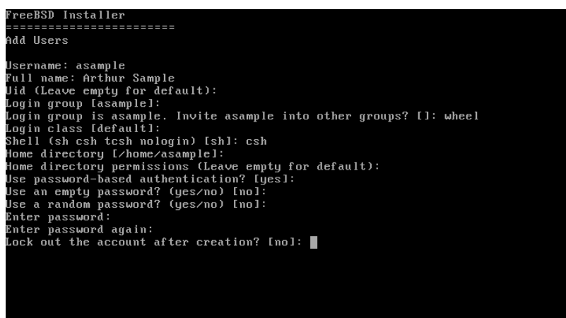
Abbildung 2.44. Benutzerinformationen eingeben
