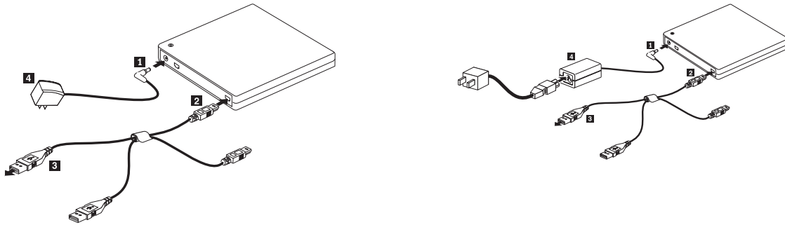
Figure 1-1. Configuration 1 : Alimentation autonome (boîtier d'alimentation)
