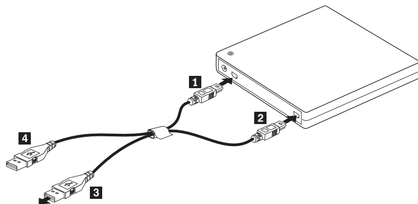
Figure 1-2. Configuration 2 : Alimentation par le bus USB standard
