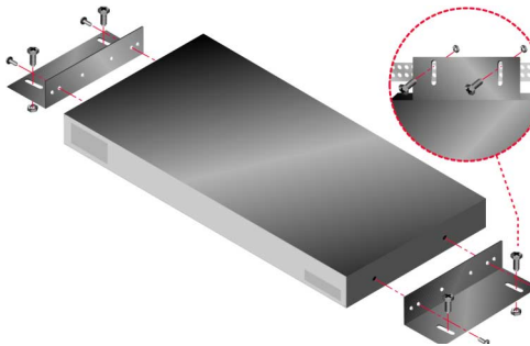
図 2.1: アプライアンスの垂直方向の設置
