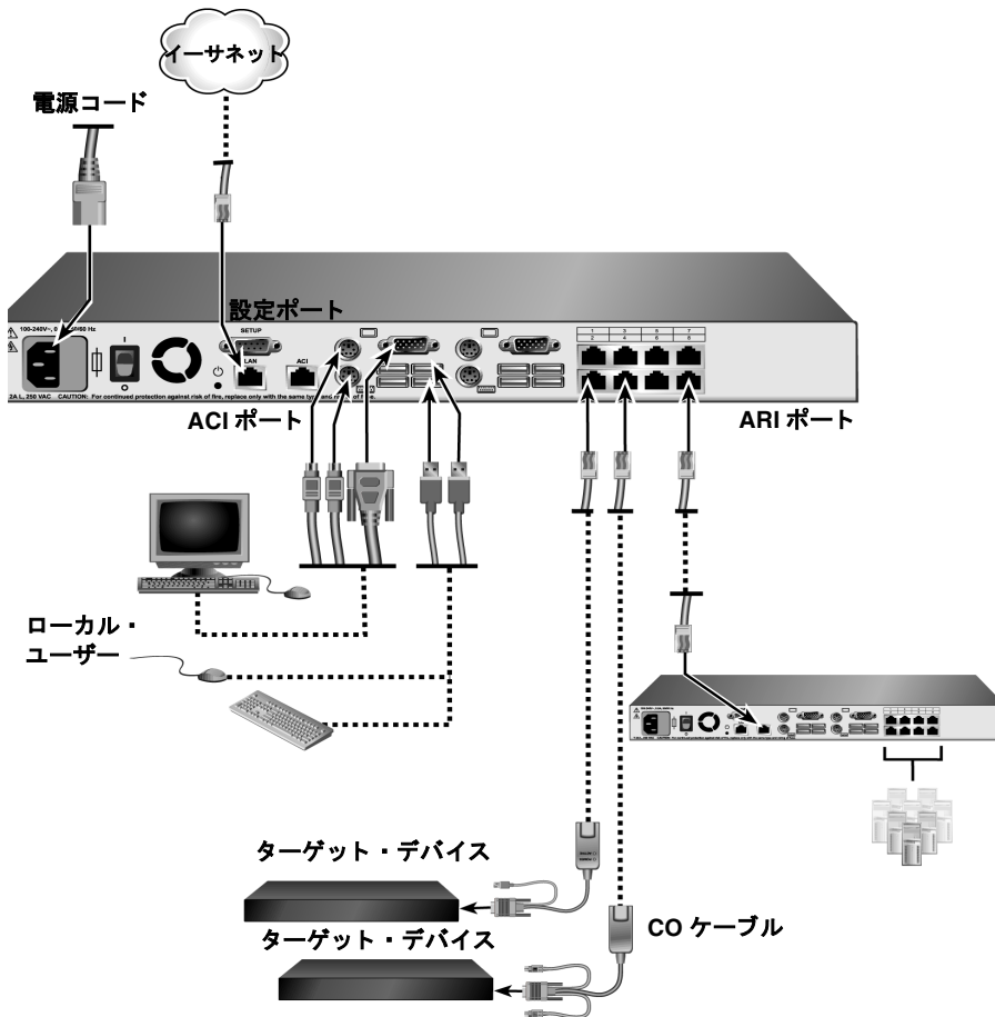
図 2.3: LCM2 アプライアンスの基本設定
