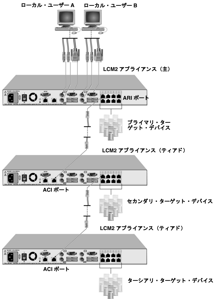
図 2.4: ティアド・アプライアンスを使用した LCM2 アプライアンスの構成
