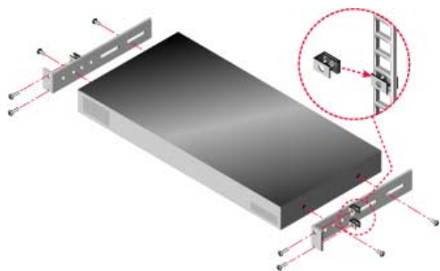
図 2.2: アプライアンスの水平方向の設置
