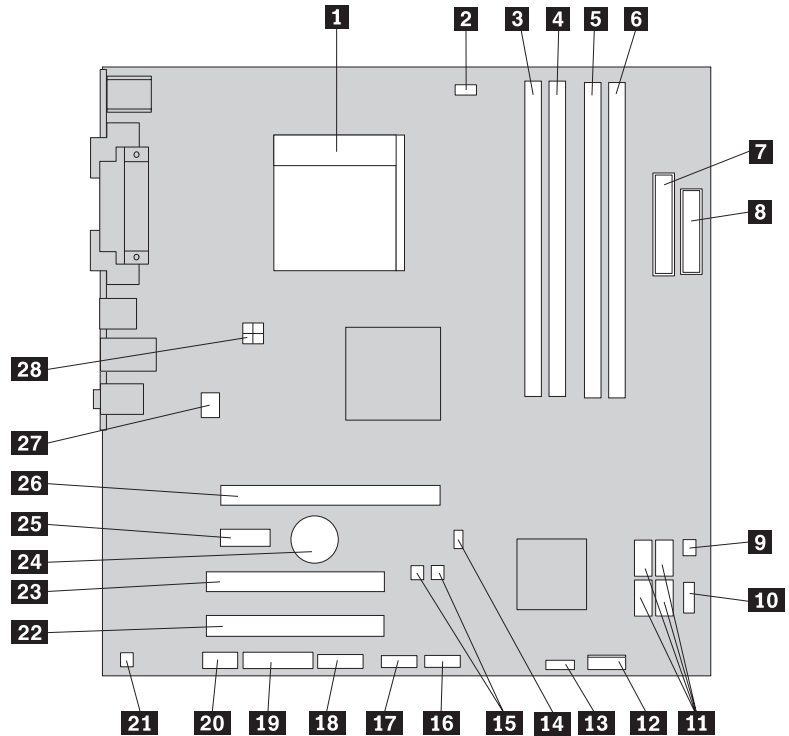
תרשים 4. מיקום חלקים בלוח המערכת
