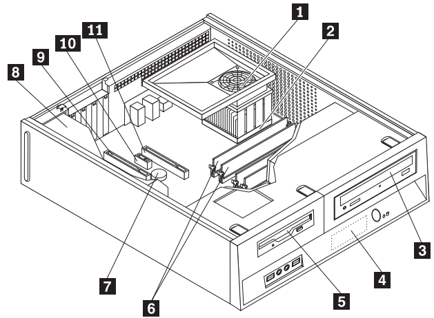
תרשים 3. מיקומי רכיבים
