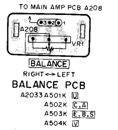
BALANCE RIGHT ↔ LEFT BALANCE PCB A2033 A501K [U] A502K [C,A] A503K [E,B,S] A504K [V]
