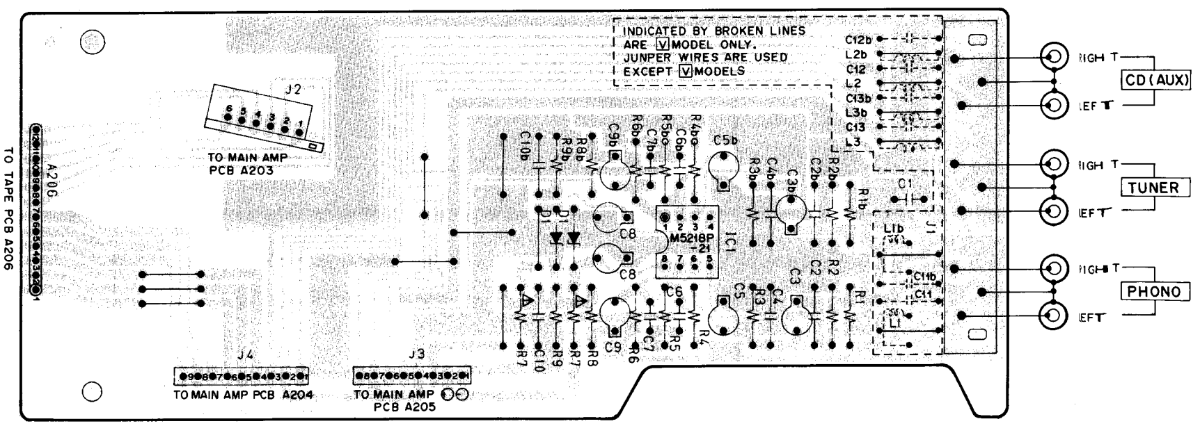
EQUALIZER PCB A2033A501B A502B C,A A503B E,B,S A504B
