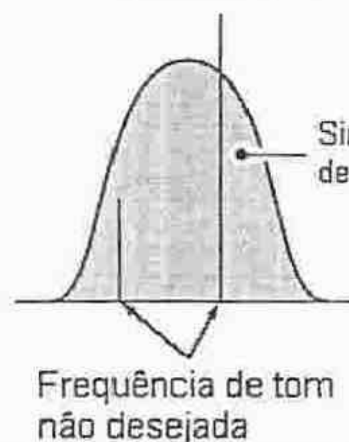
Corte Automático Desativado
