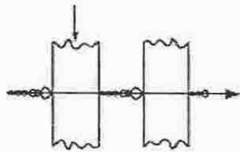
Componentes do ruído
