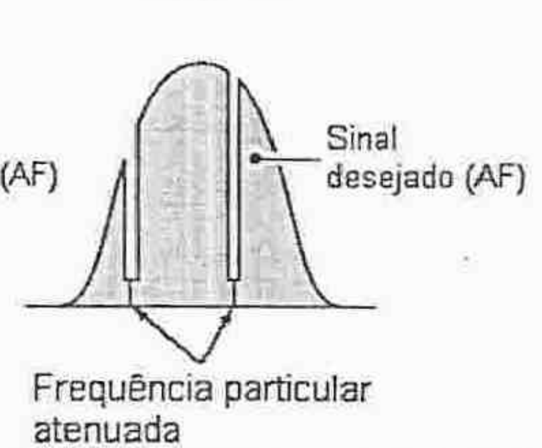
Corte Automático Ativado
