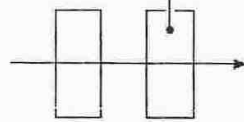
Sinal desejado (CW)
