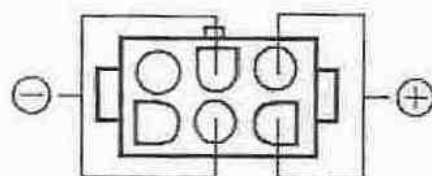
Vista do Painel Traseiro
