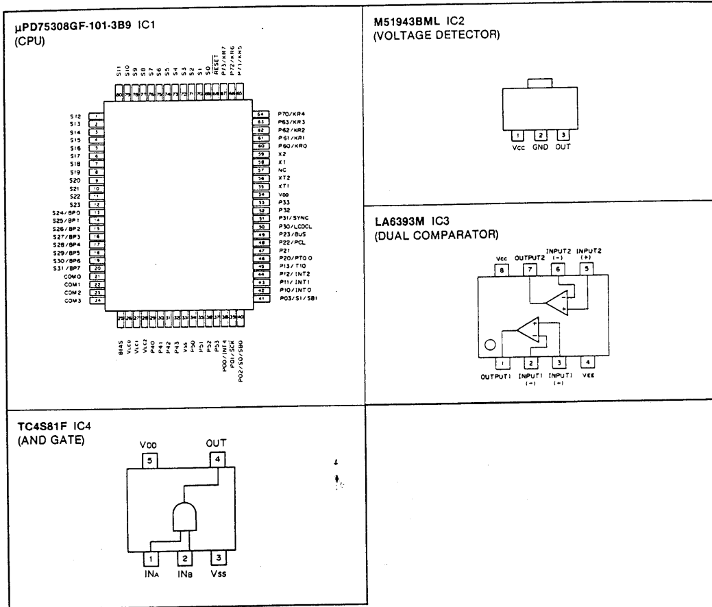
1SS184 D4, D6, D7, D9 D12 (IC-3210A/E: Europe, Australia) D22
