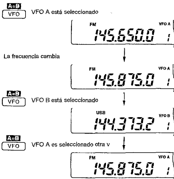
la frecuencia cambiada (145.875 MHz) aparece
