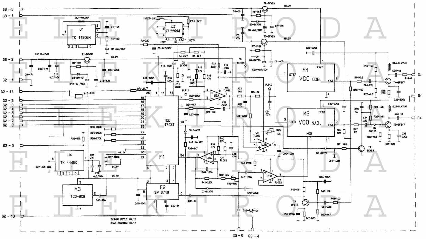
SCHEMAT BLOKU SYNTAZY 3044-8000
