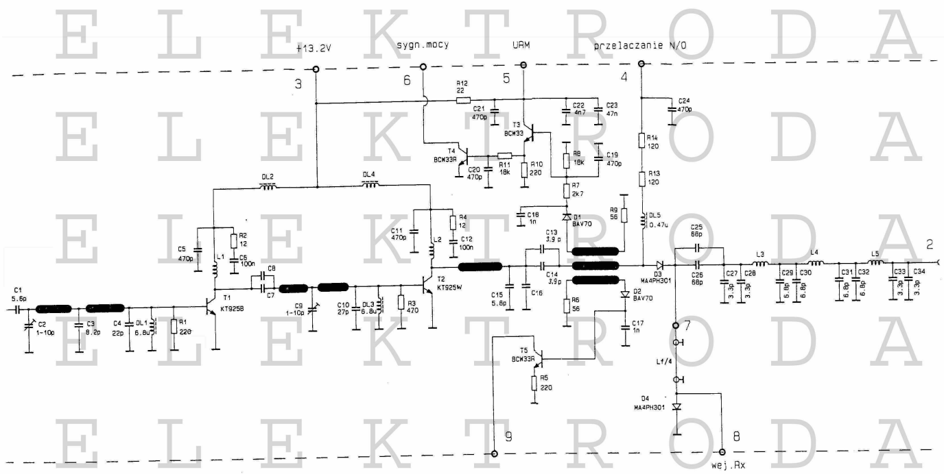
SCHEMAT BLOKU MOCY 3045-3000
