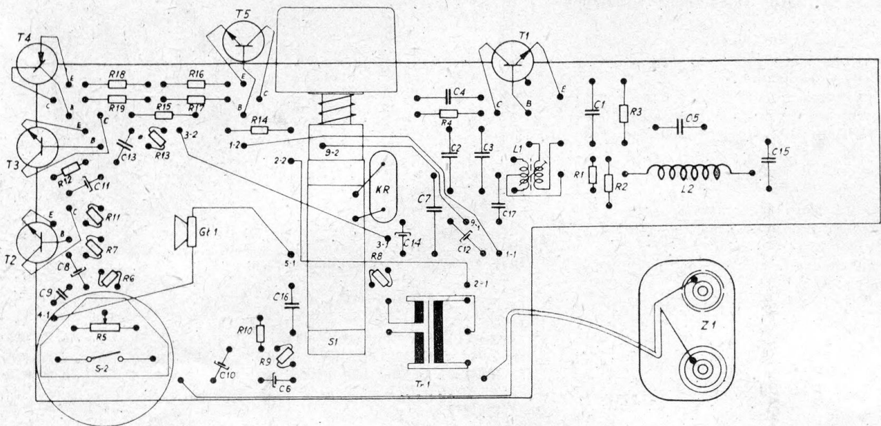
Rys. 2. Schemat ideowy radiotelefonu TROP
