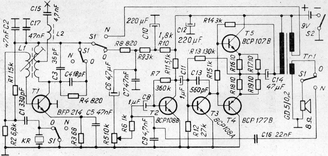
Rys. 2. Schemat ideowy radiotelefonu TROP
