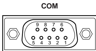
Aanzicht achterpaneel
