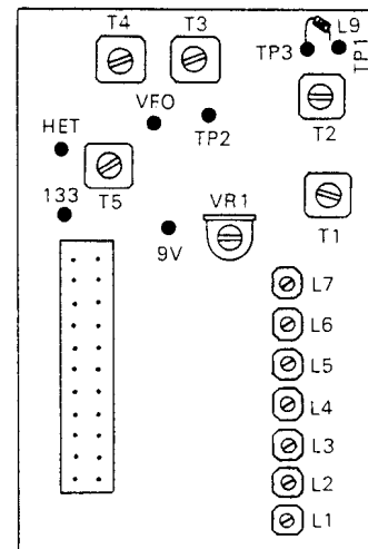
HET unit (X50-1300-20: 700A)
