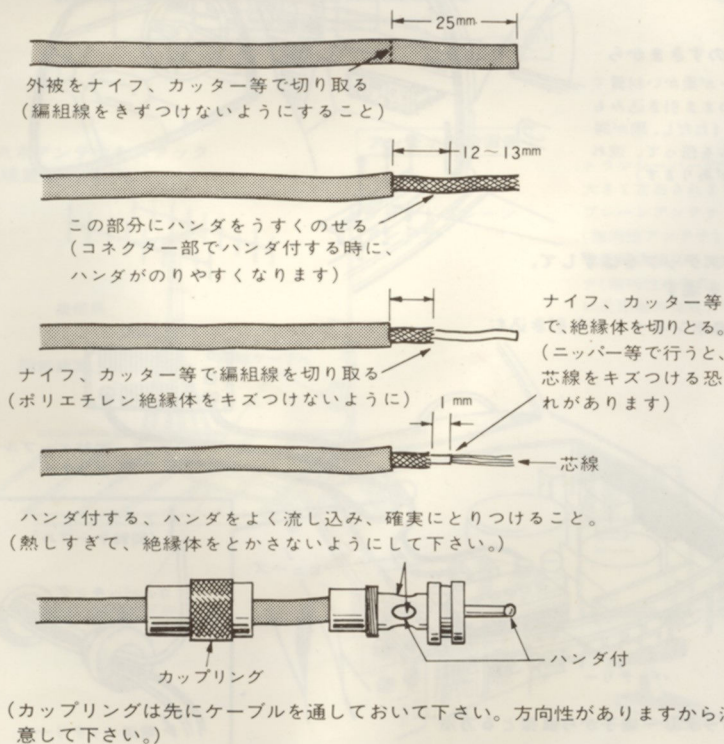
図2 M型コネクタの取り付け方
