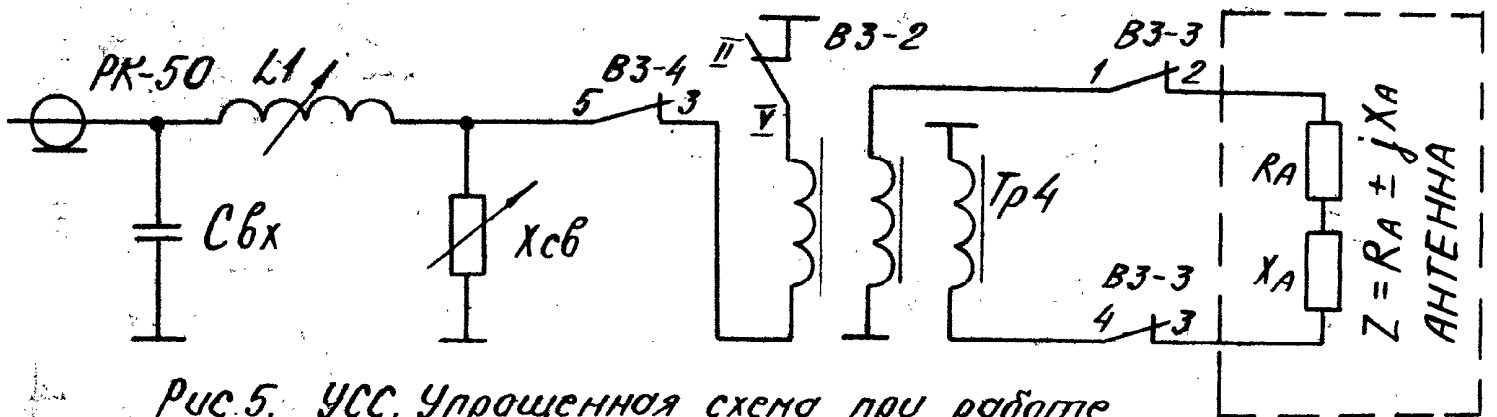
Рис. 4. УСС. Упрощенная схема при работе в диапазоне частот 1,5-4 МГц.
