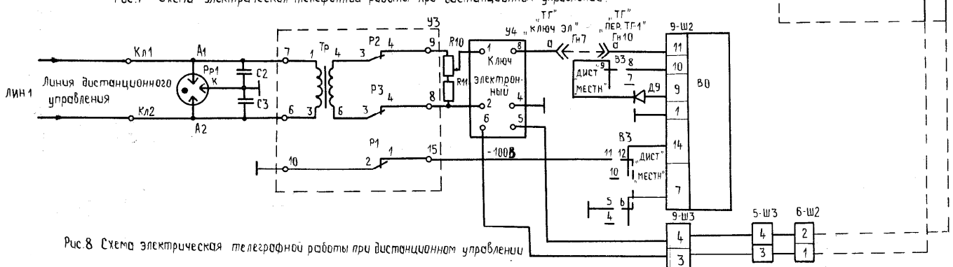
Рис.7 Схема электрическая телефонной работы при дистанционном управлении.
