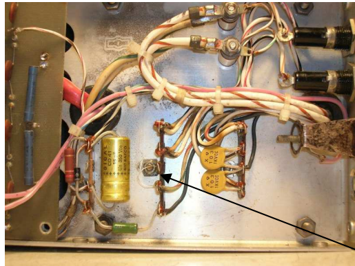
Fusible de protection des 811A
