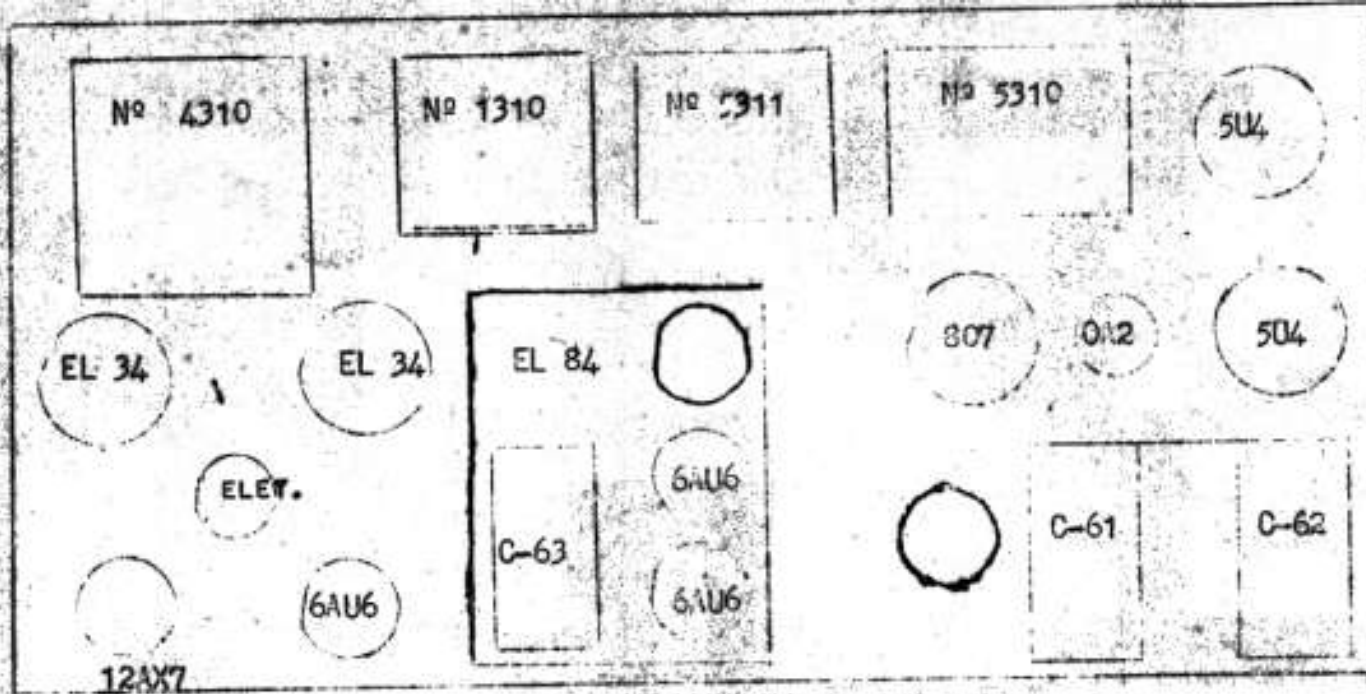
FIG. 1 - CHASSIS VISTO DE CIMA
