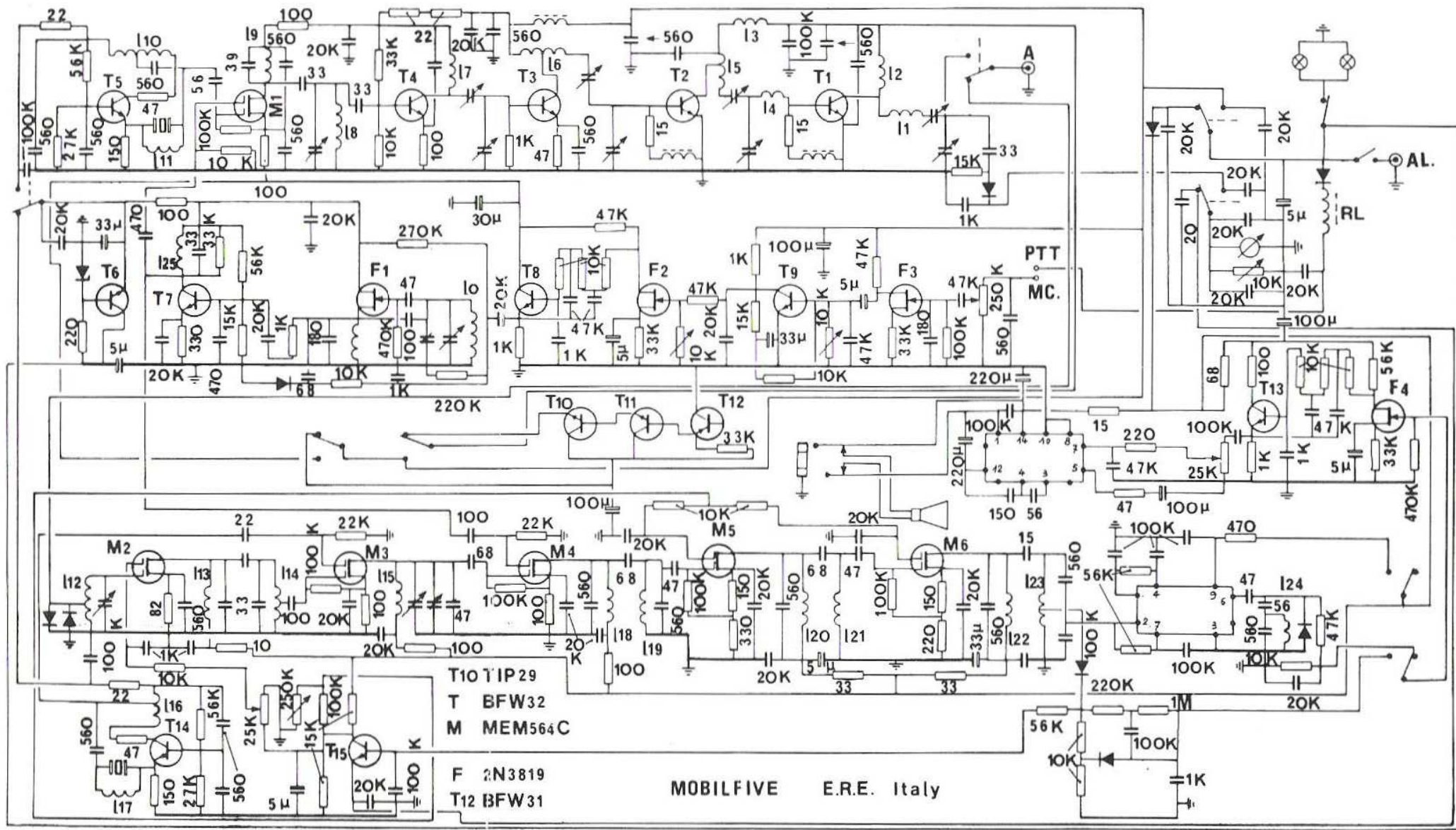
schéma complet du transceiver "MOBILFIVE"
