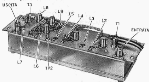
Vista superiore e inferiore del convertitore G 4/161, coi punti di taratura. Top and bottom views of G 4/161 converter, with alignment points.
