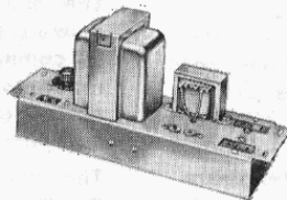
Alimentatore - AC power pack
