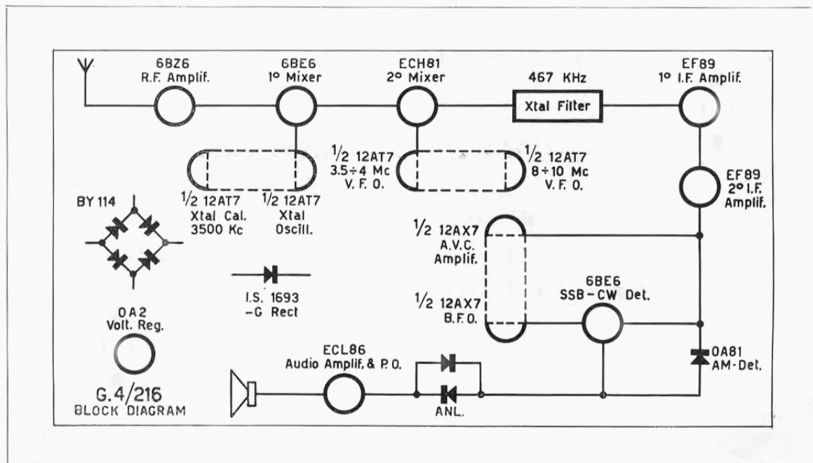
Fig. 1 - G 4/216 - Schema a blocchi
