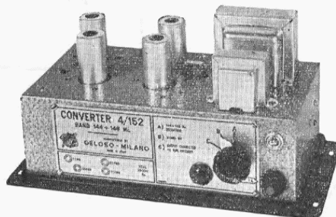
Vista posteriore del convertitore N. 4/152. Rear view of converter No. 4/152.
