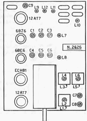
Vista superiore del Gruppo RF N. 2626.
