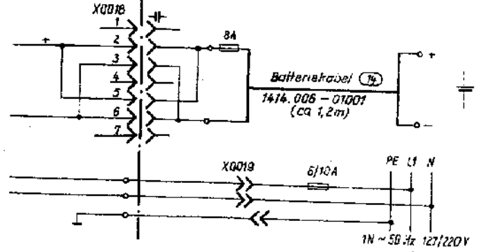
Anschlußplan 1340.042-10004 Ap
