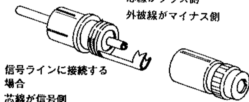
ピンプラグの接続
