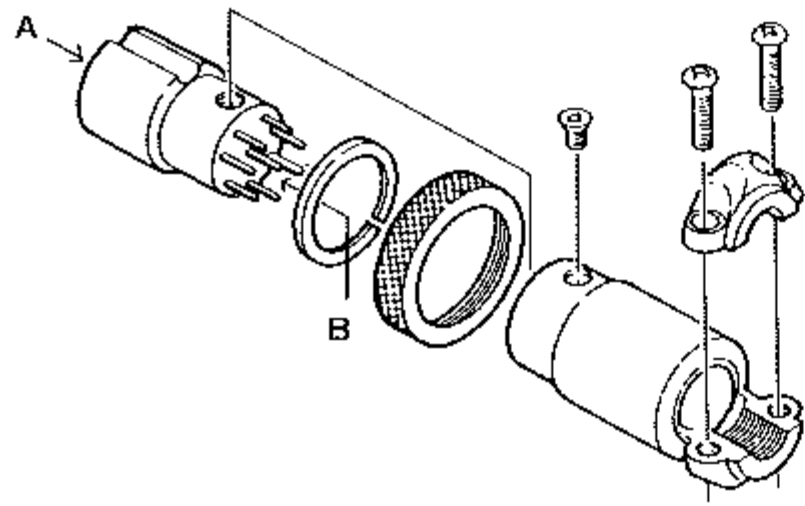
マイクロホンの接続
