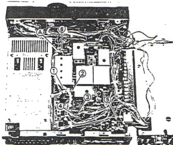
Fig. 6 connettori dell'unità locale
