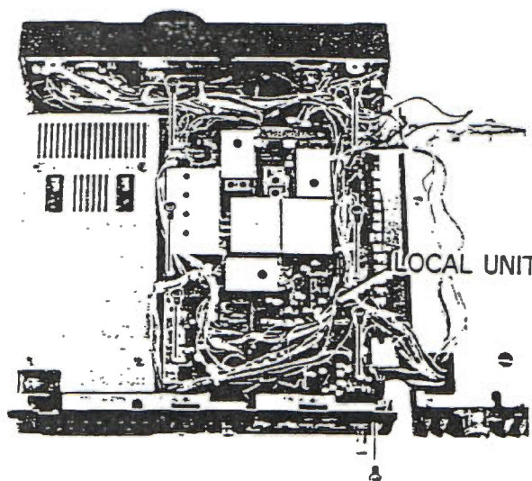
Fig.7 Viti dell'unità locale
