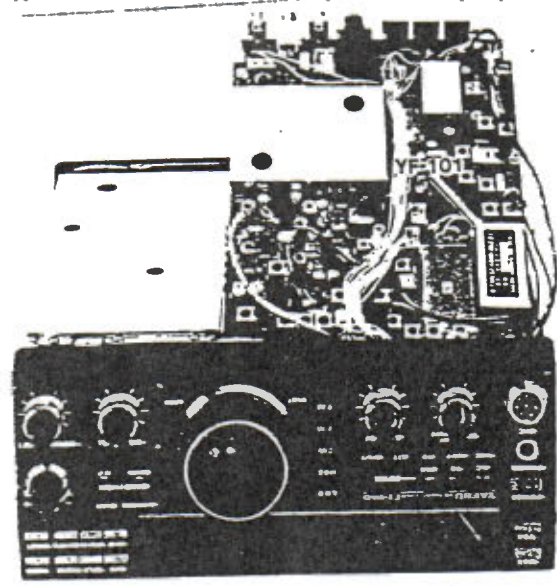
Posizione del filtro SSB
