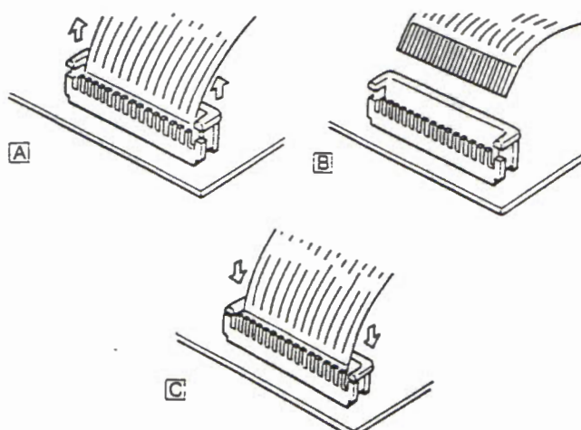
Fig. 3 connettori dei cavi piatti
