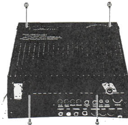
Fig. 4 rimozione del coperchio superiore
