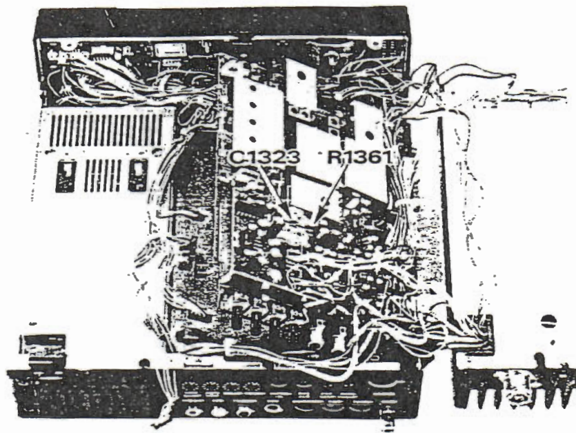
Fig.8 Componenti dell'unità locale da rimuovere
