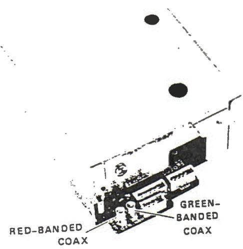
Connettori ATU-2
