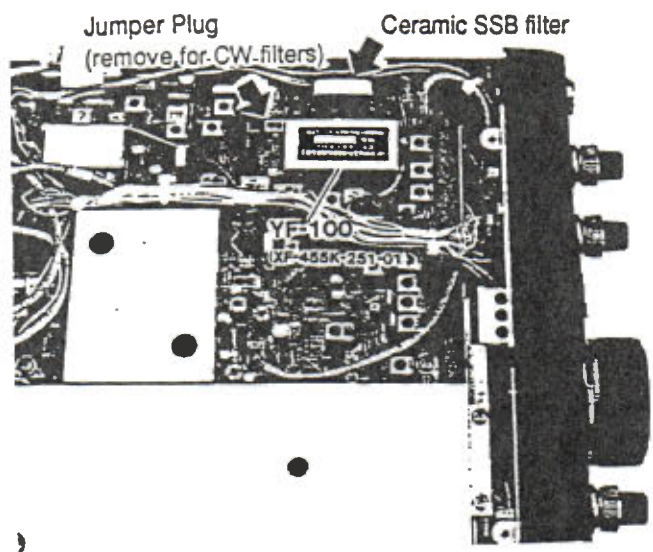
Filtro CW, ponticelli e filtro SSB ceramico
