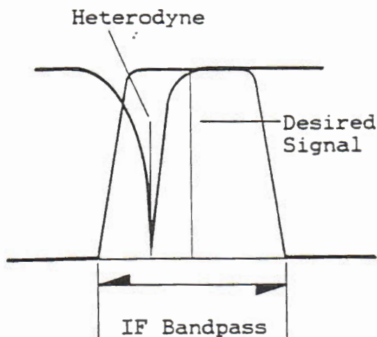
Regolazione filtro NOTCH IF
