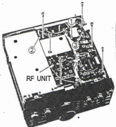
Fig. 2 posizione dell'unità RF
