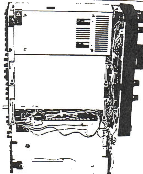
Fig. 5 Connettori dell'unità locale
