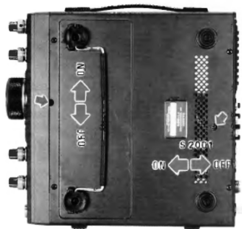
Положения выключателей на нижней крышке
