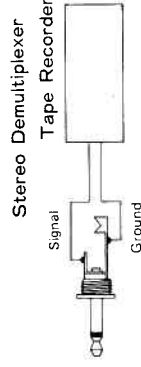
MPX. REC plug
