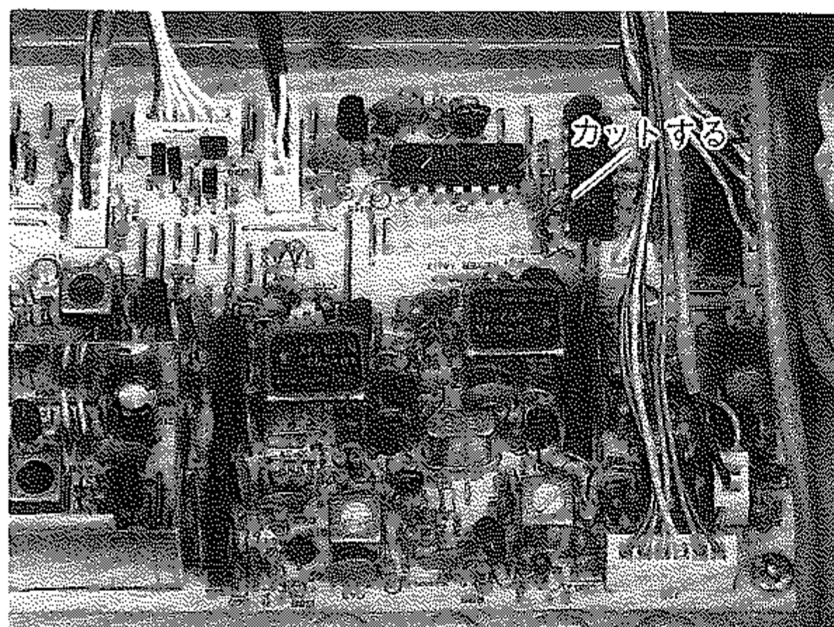
KEYER UNIT B取付前
