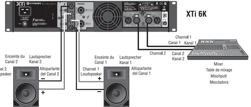
Abb. 2.6 Systemverkabelung, Stereomodus unter Verwendung der Schraubklemmen
