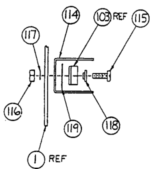
DETAIL A TYP 4 PLACES Q1, Q2, Q4 & Q6
