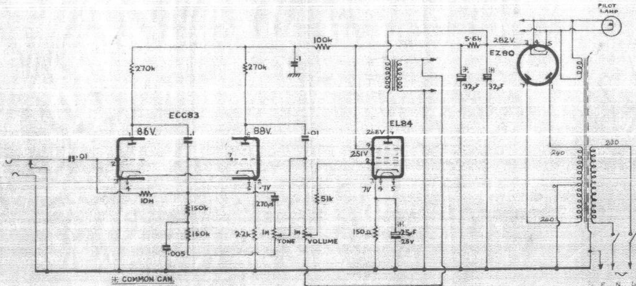
∞ CIRCUIT DIAGRAM, LITTLE GIANT, ∞ MK1
