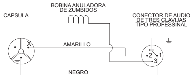
CONEXIONES INTERNAS
