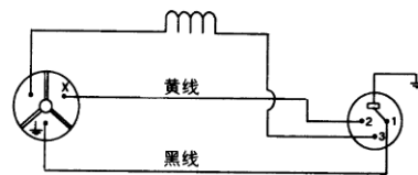
内部连接
