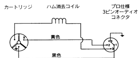
内部接続図
