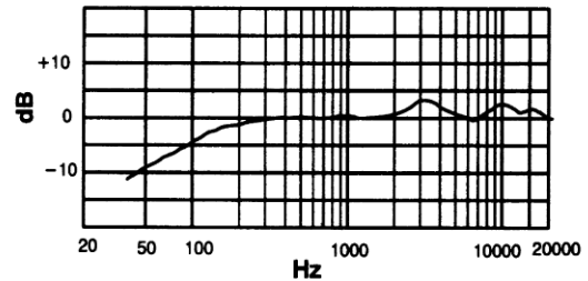
典型频率响应
