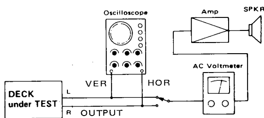
Fig. 6-4-1 Test setup for azimuth check 位相測定接続図
