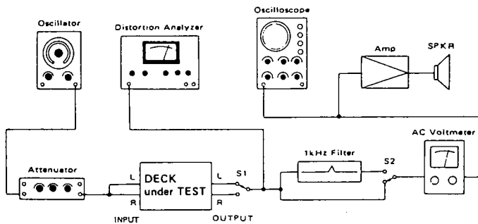
Fig. 6-8 Basic Test Setup 基本測定接続図
