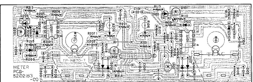
METER PCB ASSY
