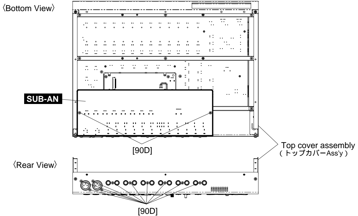
[90D]: Bind Head Tapping Screw-B (+ バインドBタイト) 3.0X8 MFZN2BL (EP600190)
