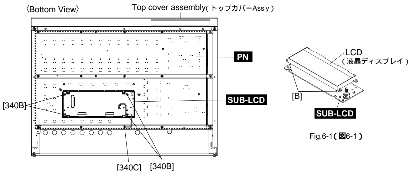
[340]: Bind Head Tapping Screw-B (+ バインドBタイト) 3.0X12 MFZN2BL (VQ074600)
