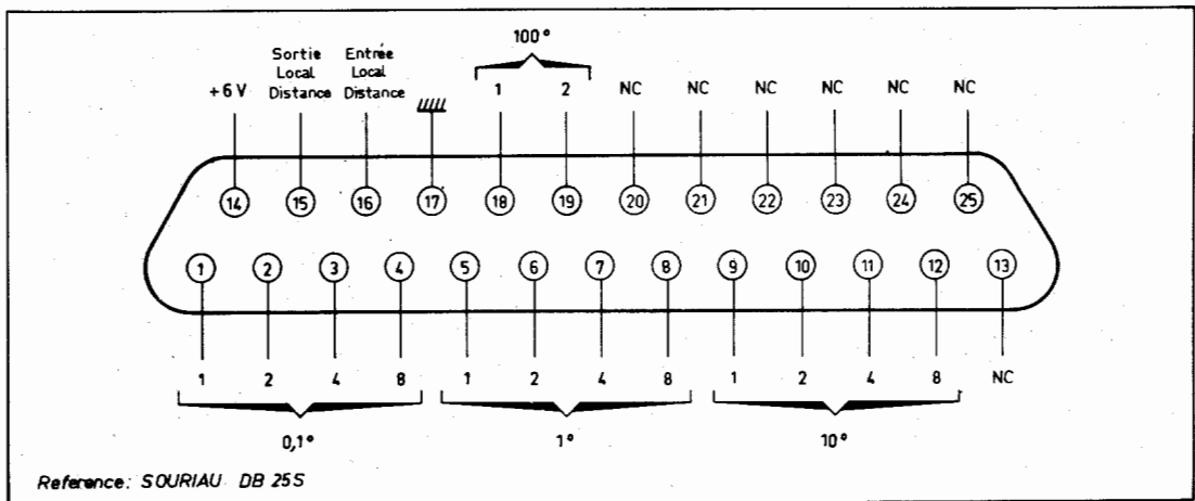
Figure V-10 CONNEXTEUR DE PROGRAMMATION (S012)
