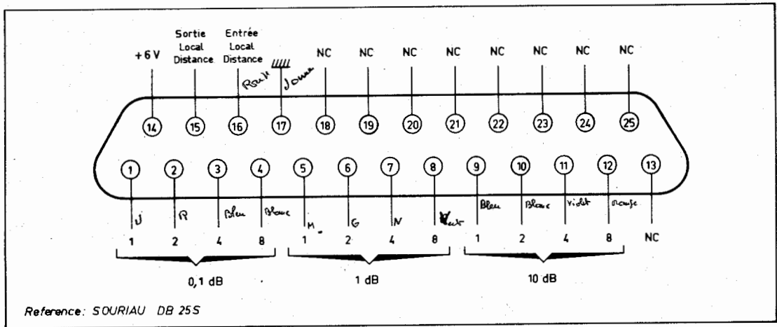
Figure V-8 CONNECTEUR DE PROGRAMMATION (S011)
