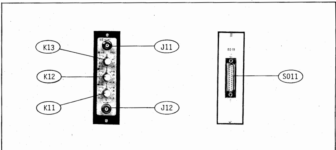
Figure V-7 OPTION ATTENUATEUR PROGRAMMABLE 3111 B
