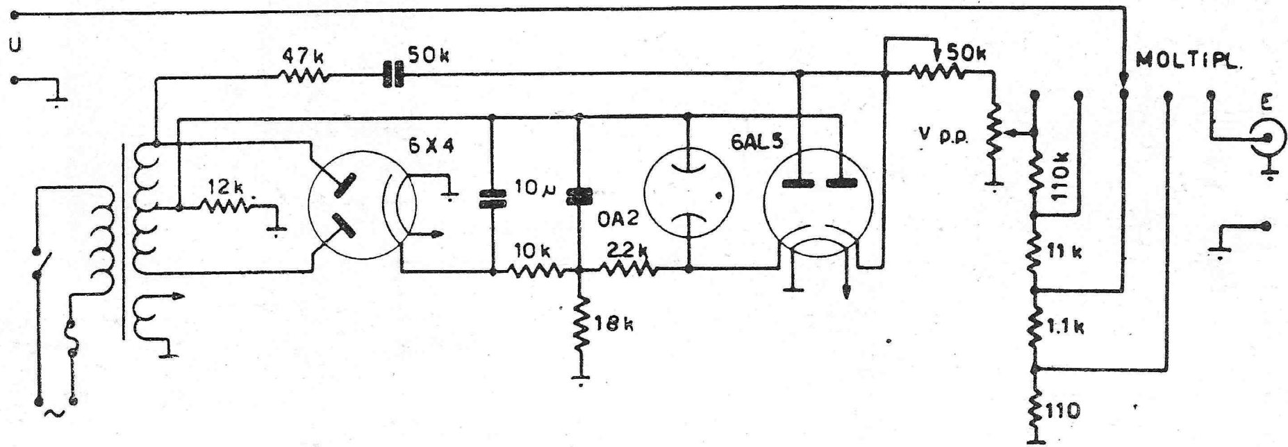
Fig. 105. - Calibratore Du Mont 264-A.
