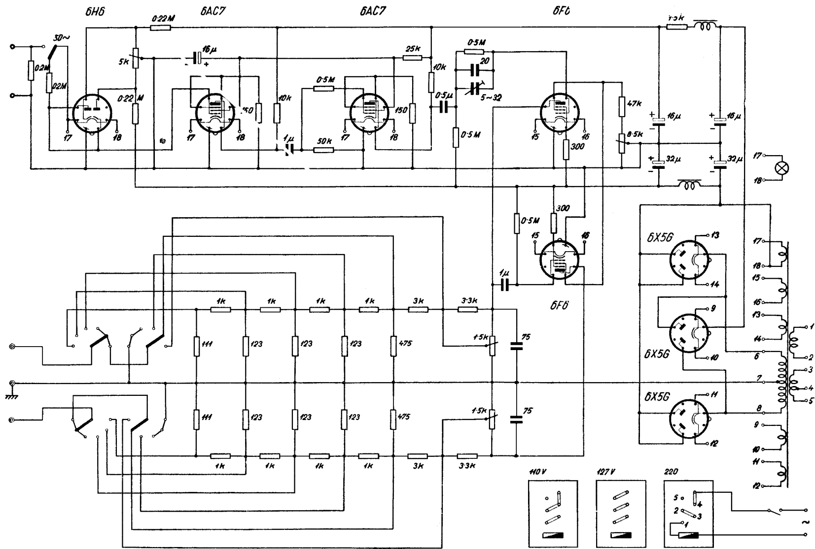
644. 49. ábra. Az EMG 1142 típusú négyszögűlámú áramforrás kapcsolási rajza
