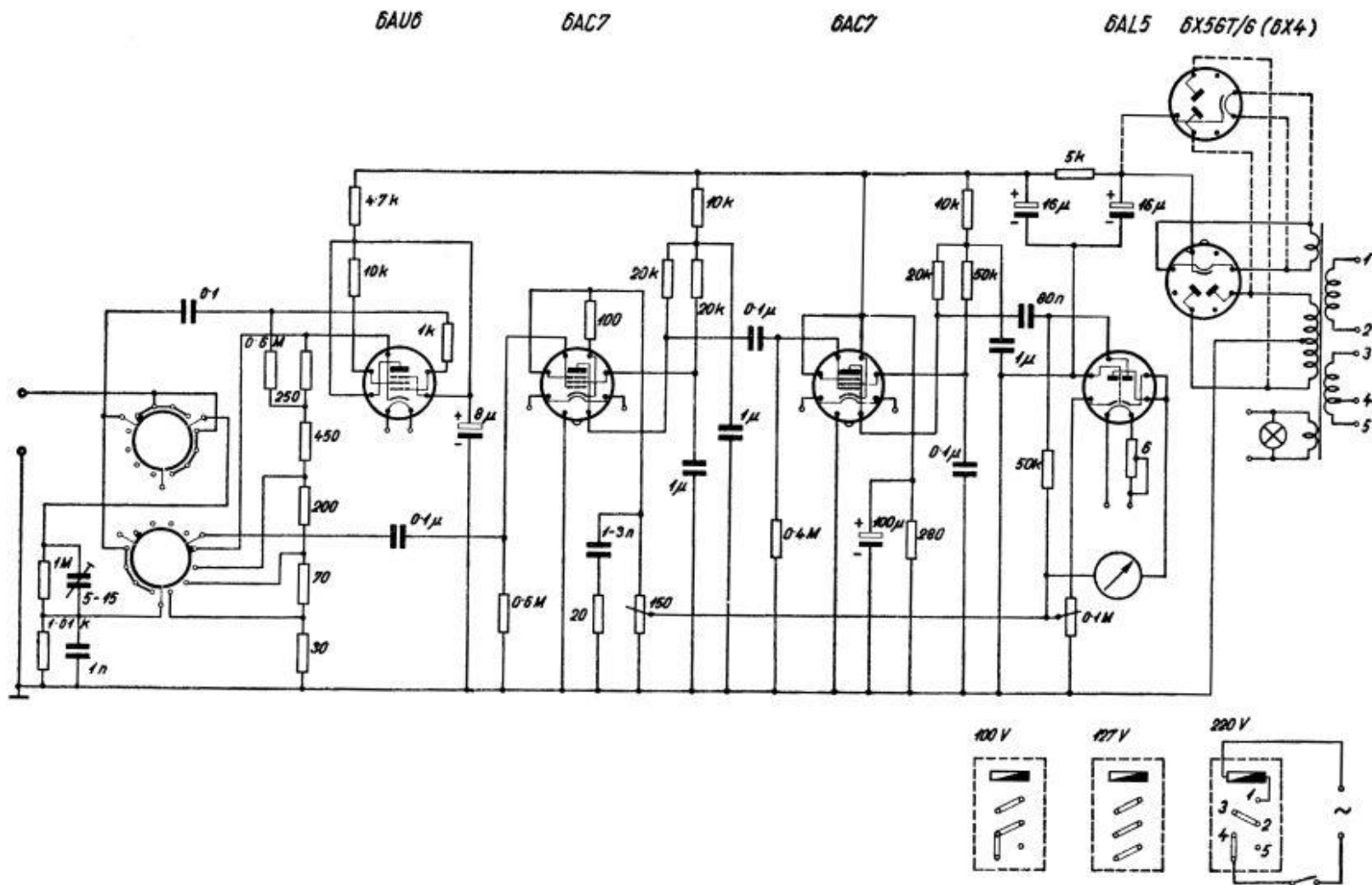
537. 85. ábra. Az EMG 1811-es esővoltmérő kapcsolási rajza
