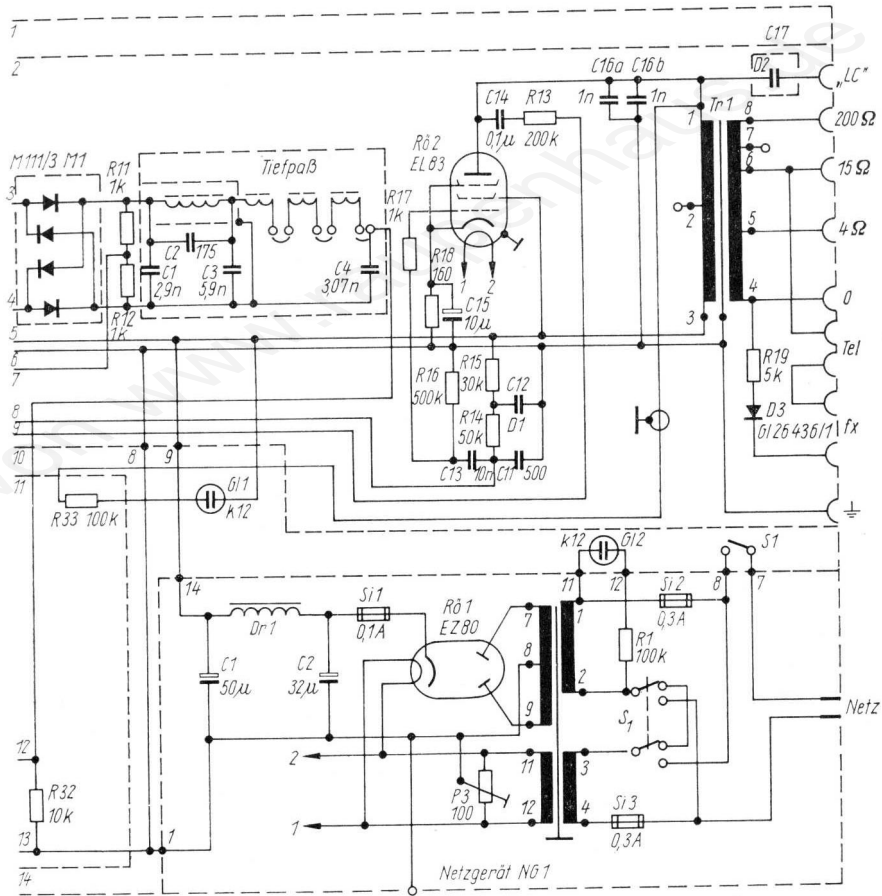
Schwebungssummer SSU 1
