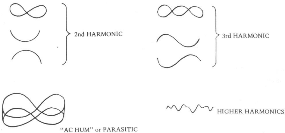
Fig. 2-3 Lissajous patterns.
