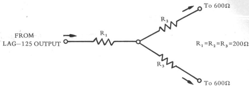
Fig. 2-7 Stereo input pad.
