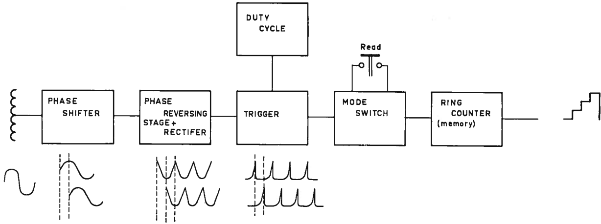
Fig. 51. Step-voltage generator
