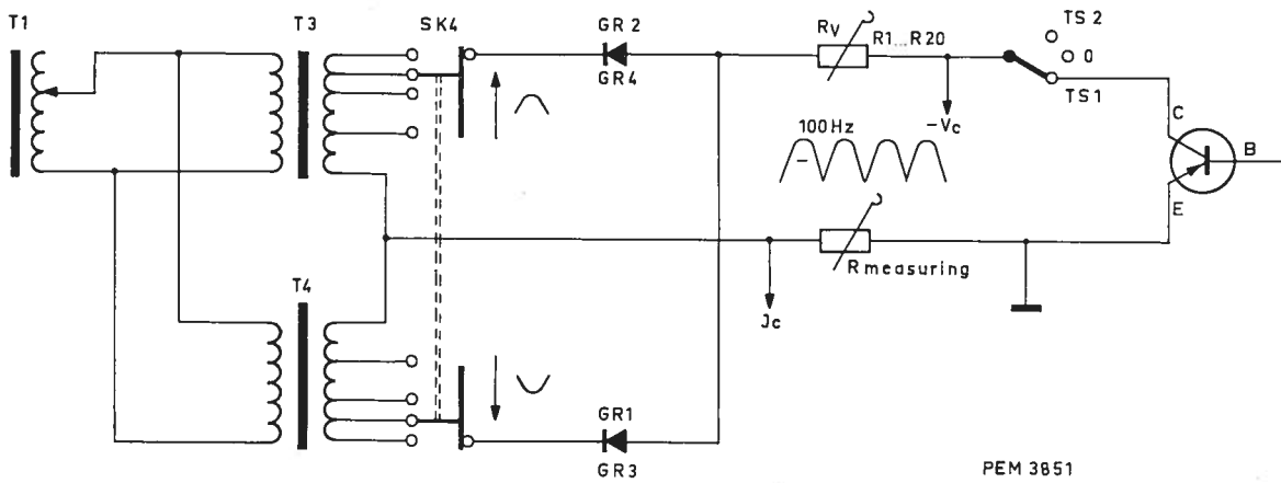
Fig. 49. Collector-voltage source
