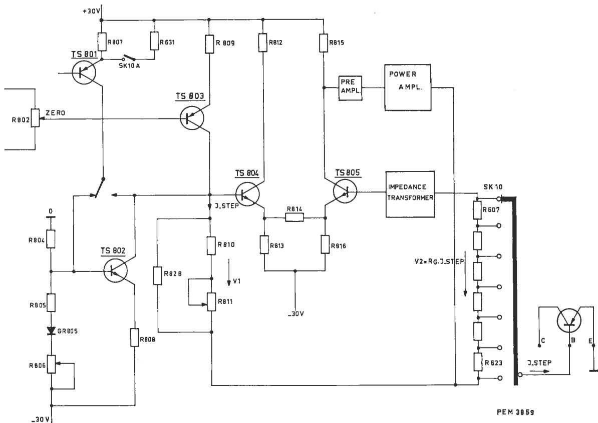
Fig. 56. Amplifier
