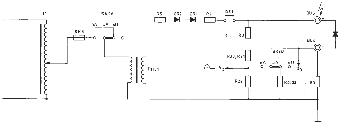
Fig. 50. H.T. source
