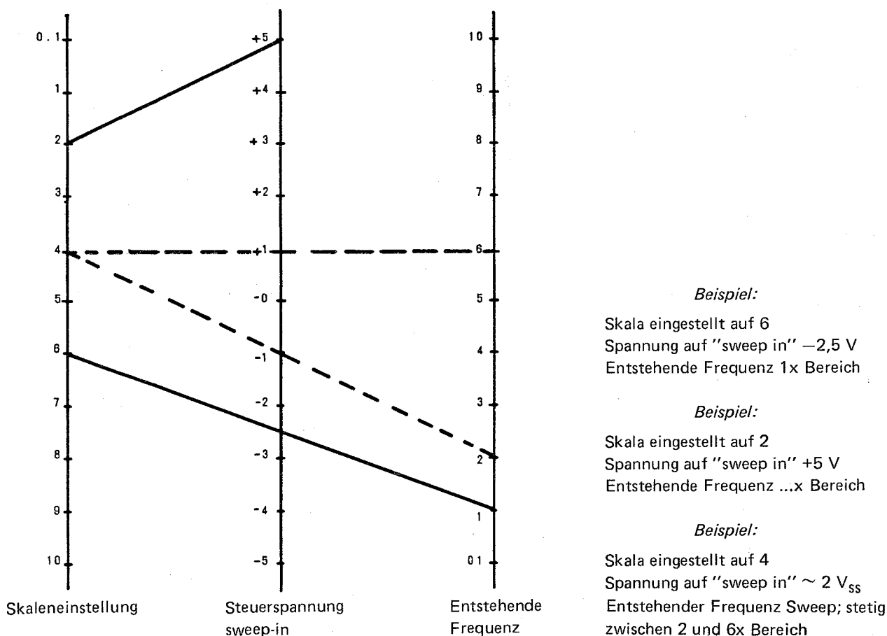
Fig. 5. Sweepbereich PM 5127
