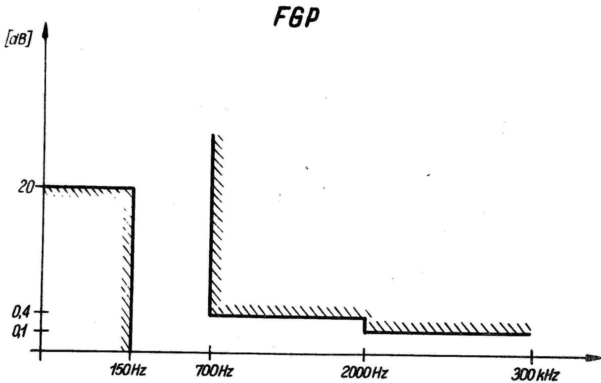
Gabaryty charakterystyk filtrów górno-(FGP) i dolno-przepustowego (FDP)
