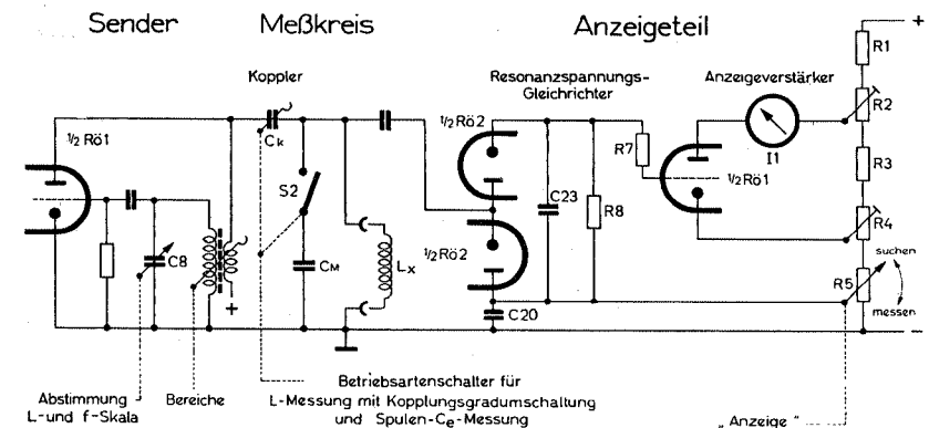
Bild 1. Vereinfachte Schaltung des L-Meßgerätes Type LARU
