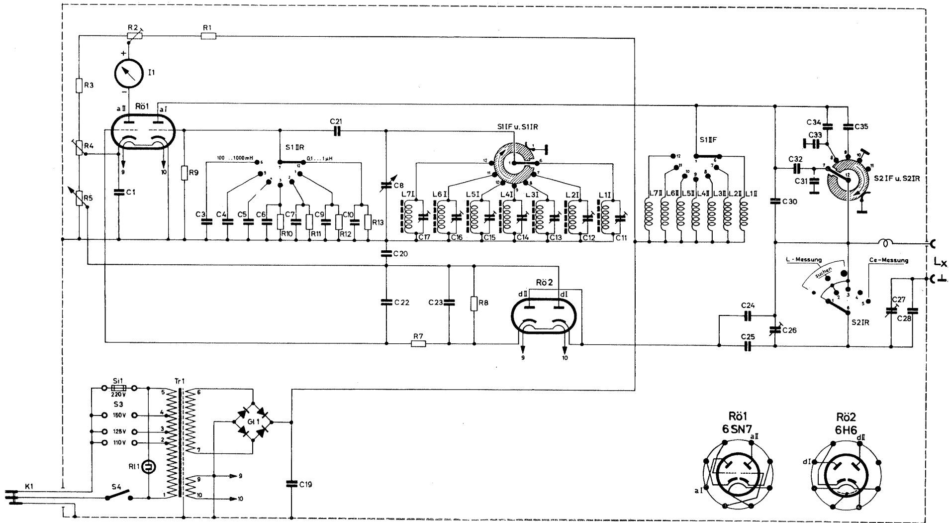
Bild 2. Stromlauf zum L-Meßgerät Type LARU BN 610
