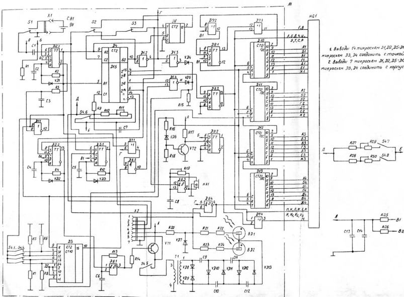
Прибор РКСБ-104. Схема электрическая принципиальная.
