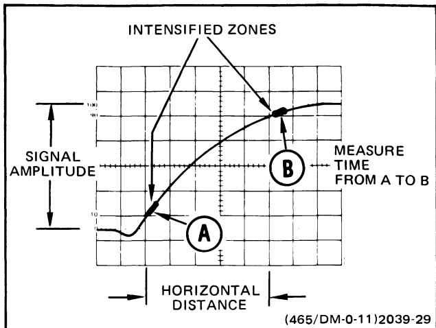
Fig. 28. Risetime.
