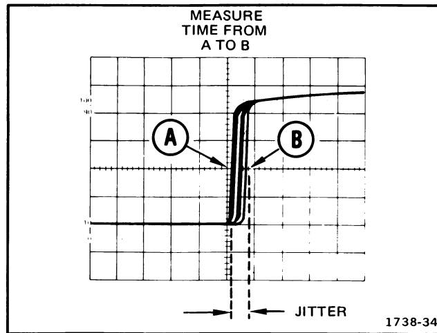
Fig. 23. Pulse jitter.
