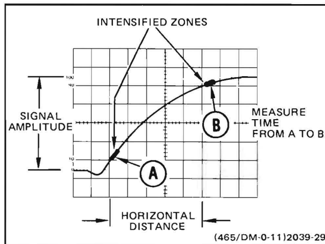
Fig. 32. Risetime.
