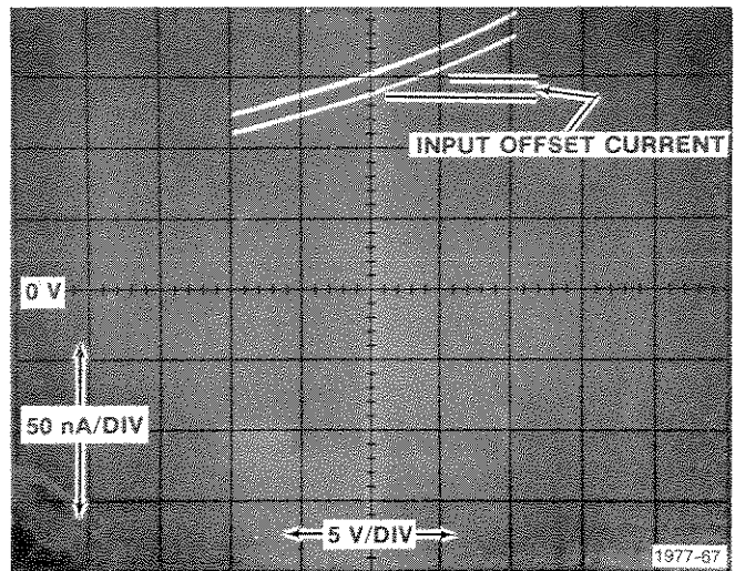
Fig. G-4. Input offset current.
