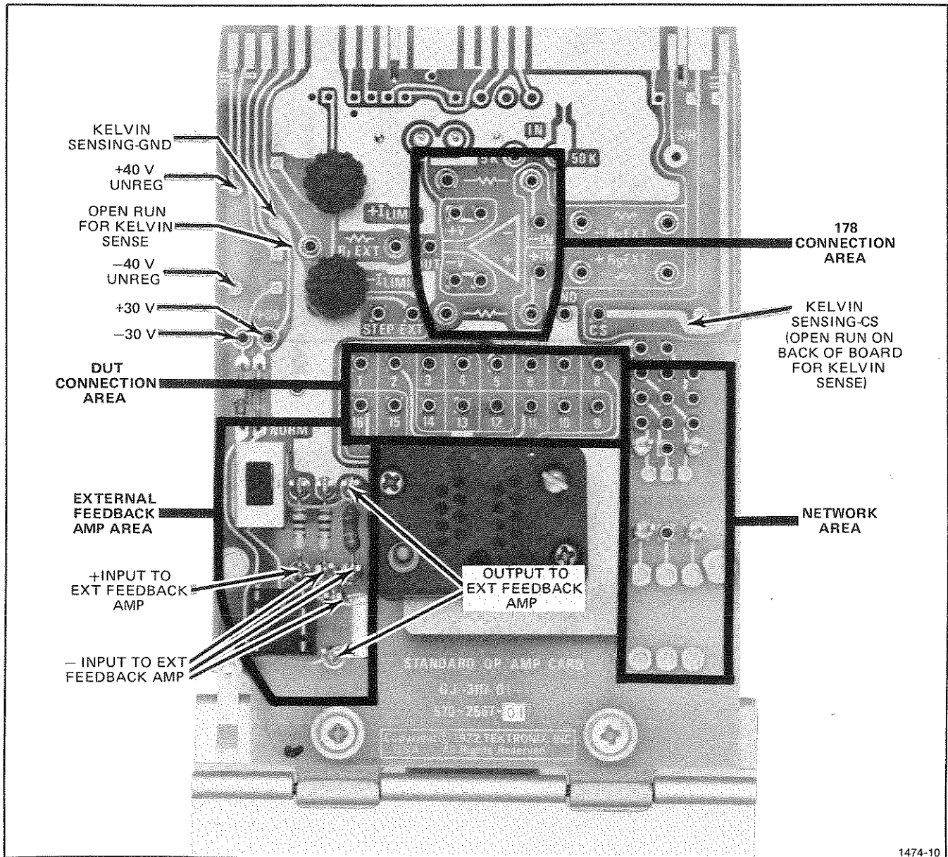
Fig. 2-9. The Standard Op Amp Card.
