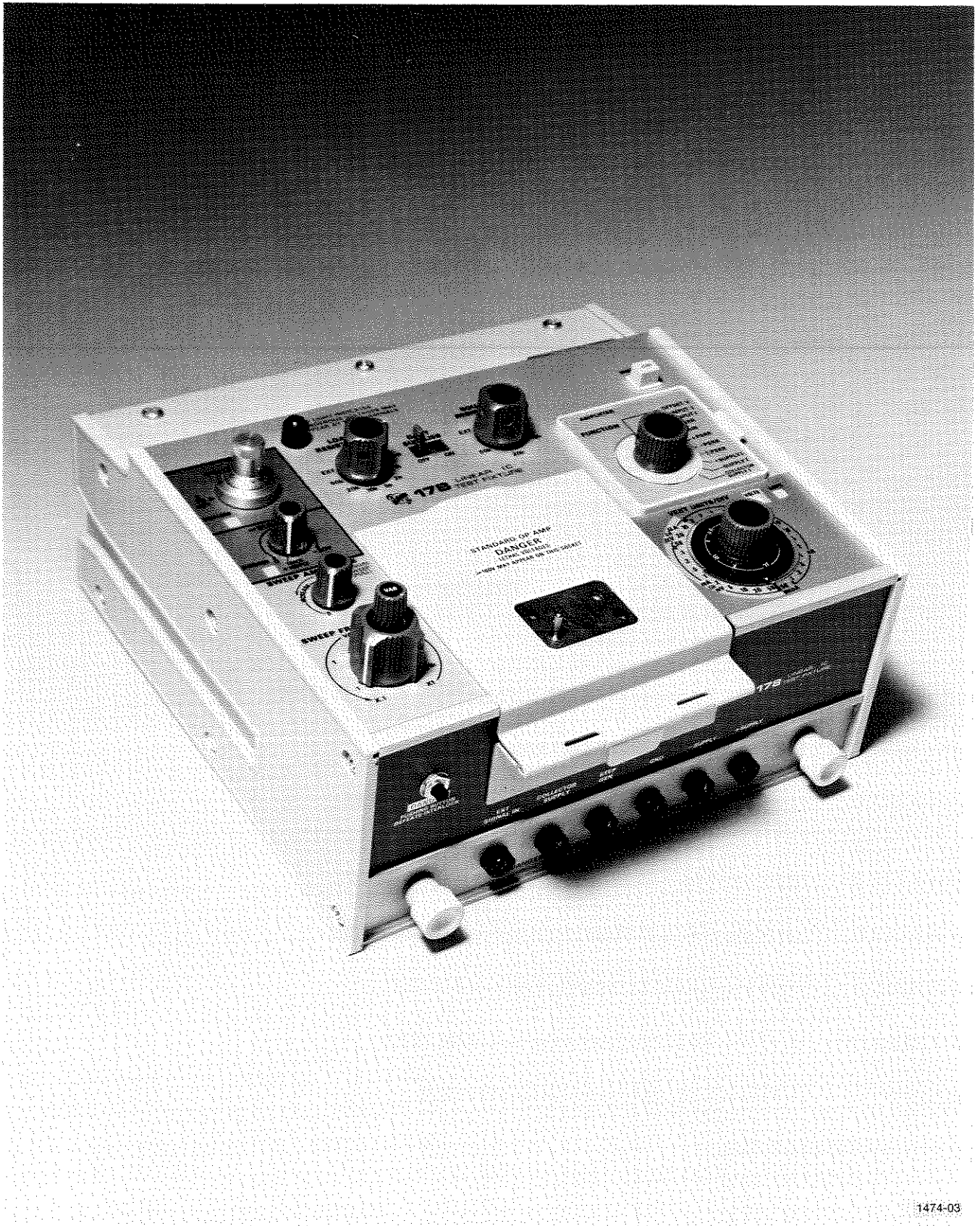
Fig. 1-1. 178 Linear IC Curve Tracer.
