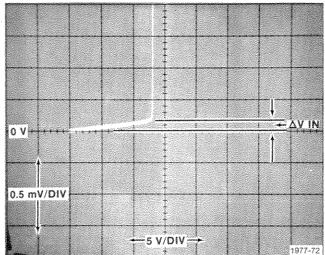
Fig. G-9. - Supply rejection ratio.
