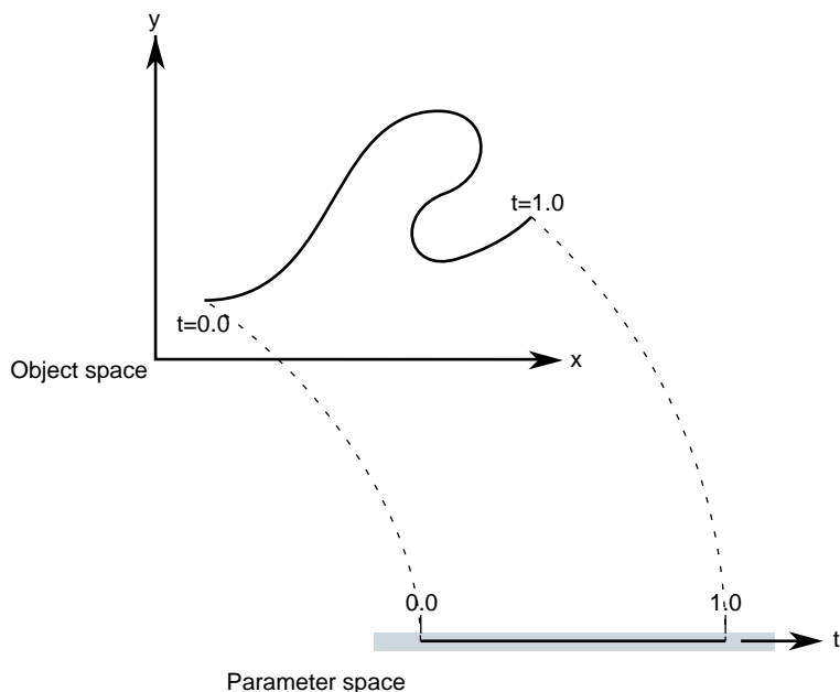
Figure 9-2 Parametric Curve: Parameter Interval (0,1).
